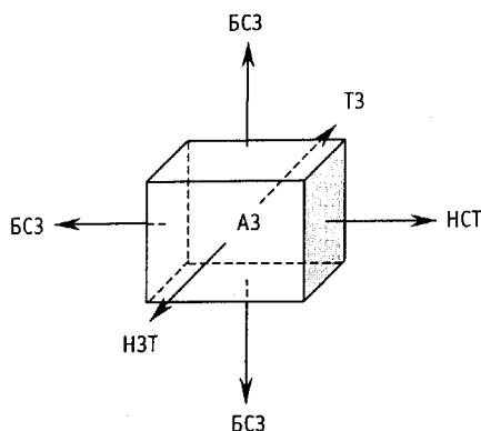
Рис. 2. Условная схема установки: НЗТ – направление вывода пучка для нейтрон-захватной терапии; НСТ – направление вывода пучка для нейтрон-соударной терапии; БСЗ – боковая сплошная защита; ТЗ – тыловая защита
